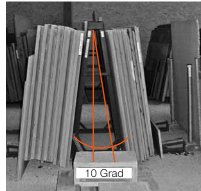
Bild 2: Gestell mit 10 Grad Neigung für die sichere Lagerung von Steinplatten.
