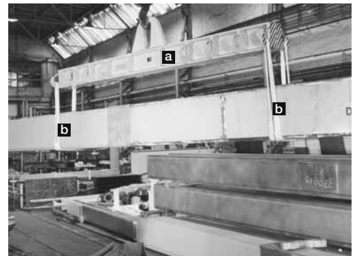
Bild 1: Einsatz des richtigen Anschlagmittels. Der Spreizbalken (a) verhindert, dass die Gurten (b) zusammenrutschen.
