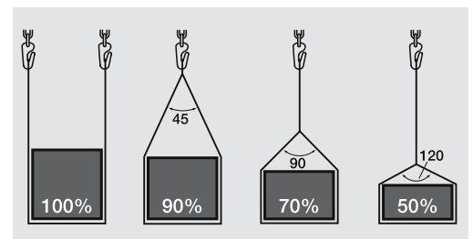
Bild 12: Einfluss des Spreizwinkels auf die Tragfähigkeit des Anschlagmittels.
